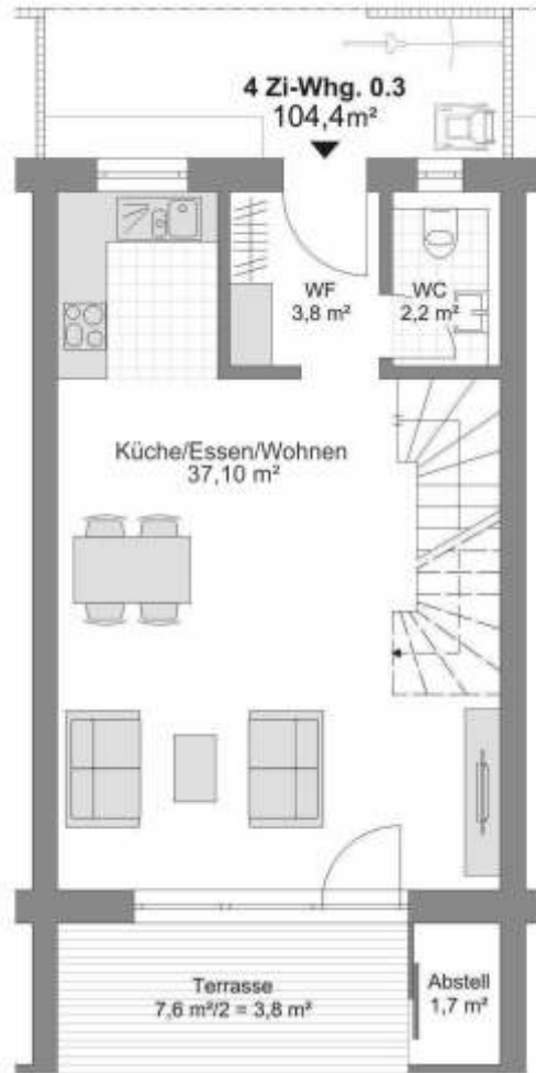
Erdgeschoss
