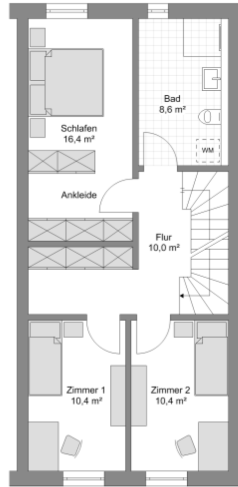
1. Obergeschoss
